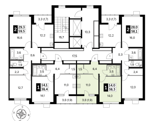
ПЛАНИРОВКА ЭТАЖА
