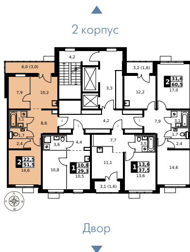
ПЛАНИРОВКА ЭТАЖА
