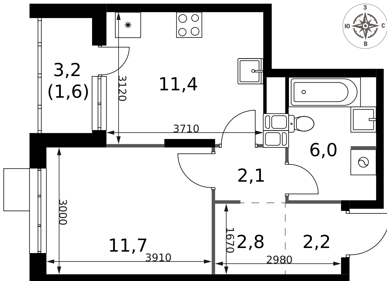
ПЛАНИРОВКА ЭТАЖА
