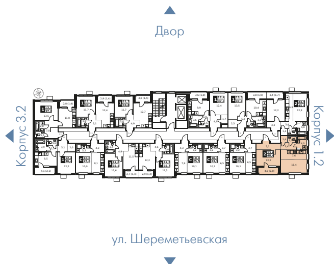
ПЛАНИРОВКА ЭТАЖА
